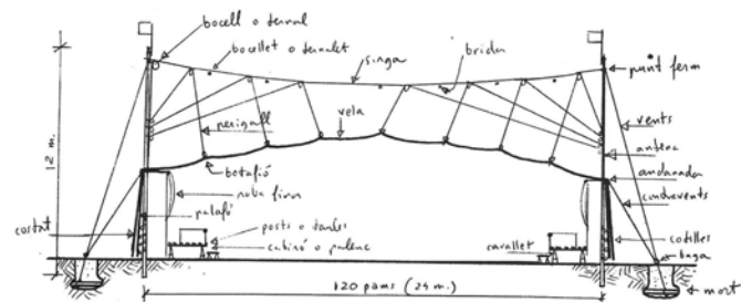
Croquis i terminologia de la secció transversal d'un envelat dibuixada per Alexandre Cirici Pellicer (1972) (ARXIU «SERRA D'OR»)
